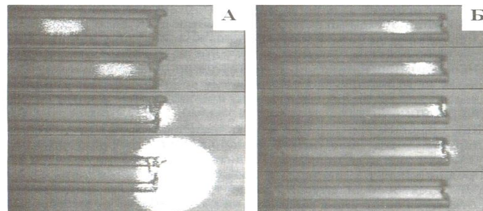
Рис. 3.8. Распространение волны в стеклянном капилляре в реакции Белоусова-Жаботинского. Химический состав БЖ реакции внутри капилляра и снаружи одинаков. Волна инициировалась на дальнем левом конце капилляра. Снимки на левой (А) и правой (Б) панелях сделаны через 5-секундные интервалы времени. Внутренний диаметр капилляра 160 мкм. (А) Общий размер = 1.45 мм × 0.71 мм, [\text{BrO}_3^-] = 0.15 \text{ M} . (Б) Общий размер = 1.9 мм × 0.44 мм, [\text{BrO}_3^-] = 0.10 \text{ M} . Концентрации других реагентов БЖ-реакции: [\text{H}_2\text{SO}_4] = 0.14 \text{ M} , [\text{MA}] = 0.02 \text{ M} , [\text{катализатор}] = 9 \times 10^{-4} \text{ M} (катализатор = сульфобатоферроин). Рисунок воспроизводится с любезного разрешения Kenneth Showalter 34
